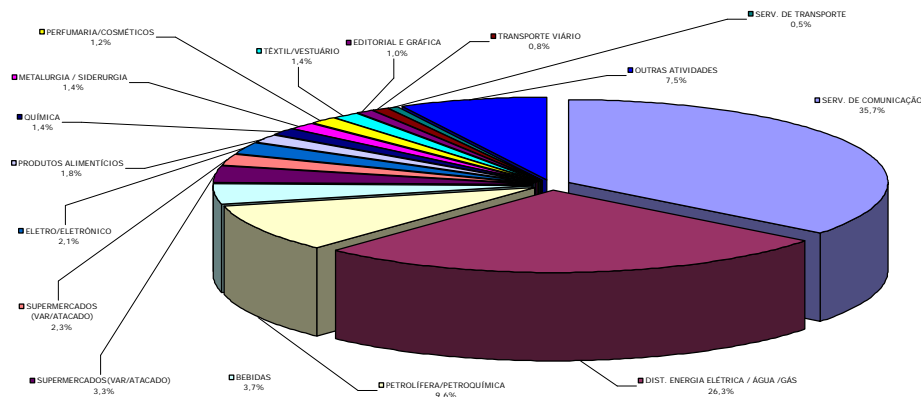
ARRECADÇÃO DO ADICIONAL DE ICMS - FECP (Lei n.º 4.056/2002) Representação percentual das principais atividades econômicas Janeiro-dezembro/2006
